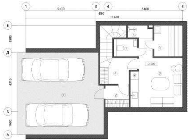
План расположения мебели и оборудования -1 этаж
