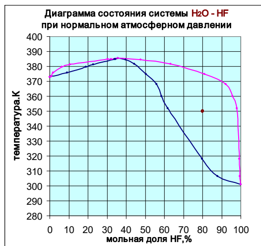
Рисунок. Диаграмма состояния системы \text{H}_2\text{O} - \text{HF}
