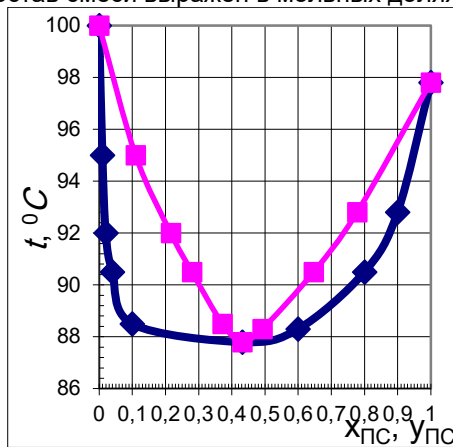
Рисунок. Диаграмма состояния системы \text{C}_3\text{H}_8\text{O} - \text{H}_2\text{O} ( P=101,3\text{Па} )
